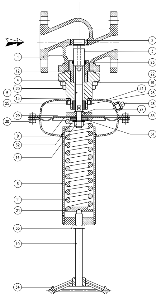
EP615 E (équilibré) avec actionneur type B, 175 cm 2
