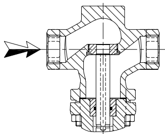
EP615 avec corps manchons taraudés
